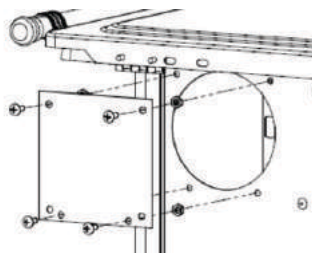
INSTALAÇÃO CORRETA
