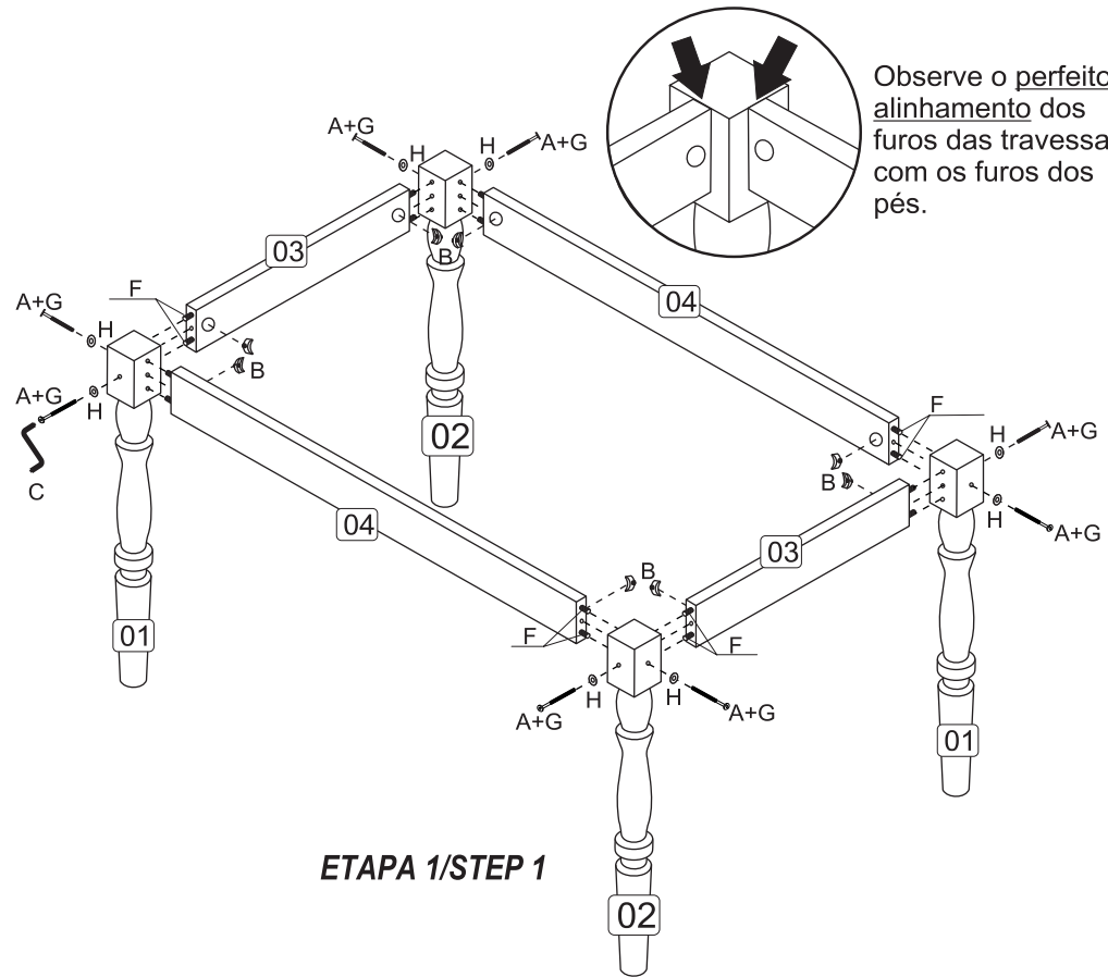
Mesa Oitavada Pés torneados
