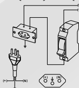
Ligação monofásica 20 A (127 V) / 10 A (220 V)
