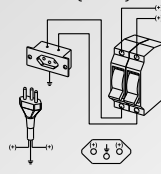
Ligação bifásica (220 V)
