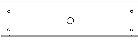
5 (15 x 133 x 470mm)-4x (0,59 x 5,24 x 18,50in)
