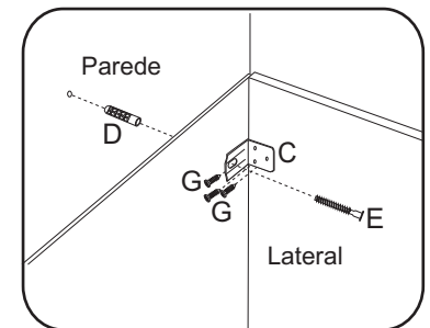
Fixação na parede
