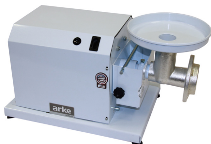
Moedor/extrusor completamente montado
