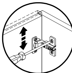
Regulagem Vertical Ajuste Vertical
