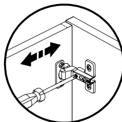
Regulagem Horizontal Ajuste Horizontal
