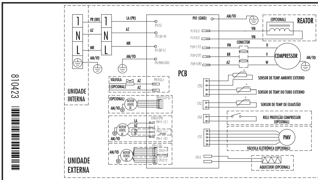
Diagrama Condensadora para os modelos 9000 - 12000 BTUs.
