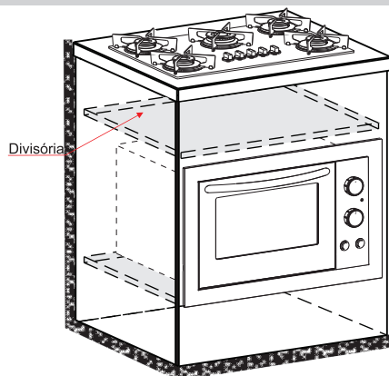
Corte lateral do nicho Ilustração cooktop com forno
